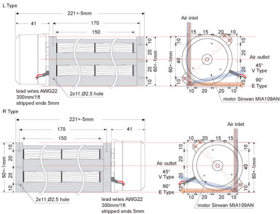
Motor Sinwan Motor MIA109AN
