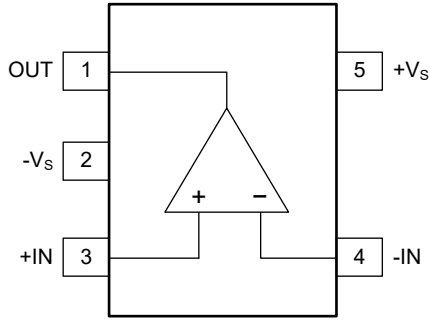
SOT-23-5
