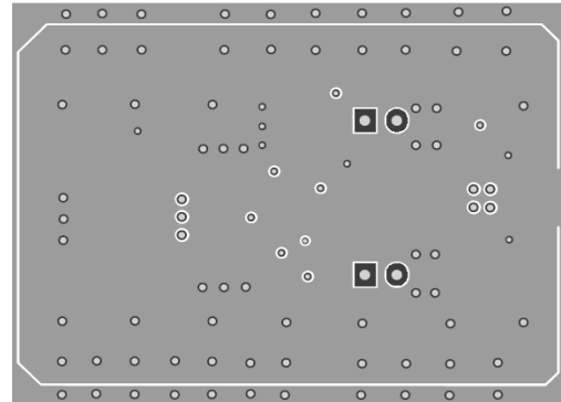
Inner Layer 1
