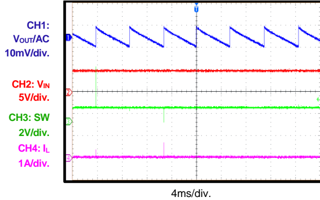
V_{OUT} Ripple
