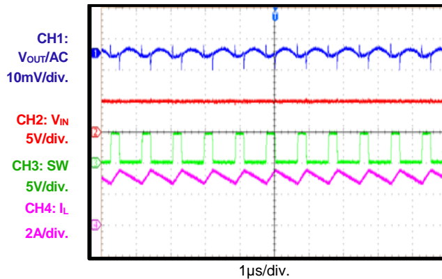
V_{OUT} Ripple
